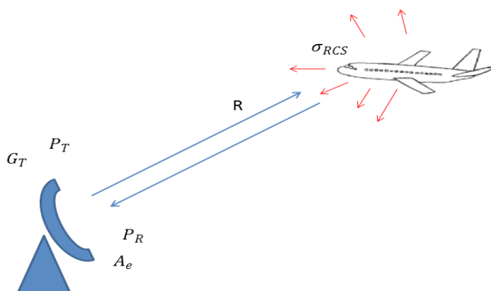
Figura 1 – Descripción del uso de la Ecuación Básica Radar Fuente: Fundamentos de un Sistema radar INDRA
