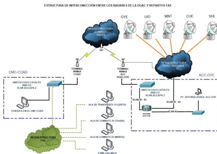
Figura 3 – Diagrama de red de la solución propuesta Fuente: Elaboración propia
