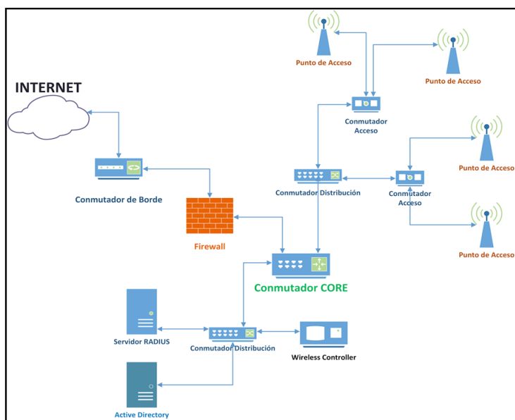
Figura 2 – Topología de una red inalámbrica para el acceso a Internet (Narváez D., 2017)
