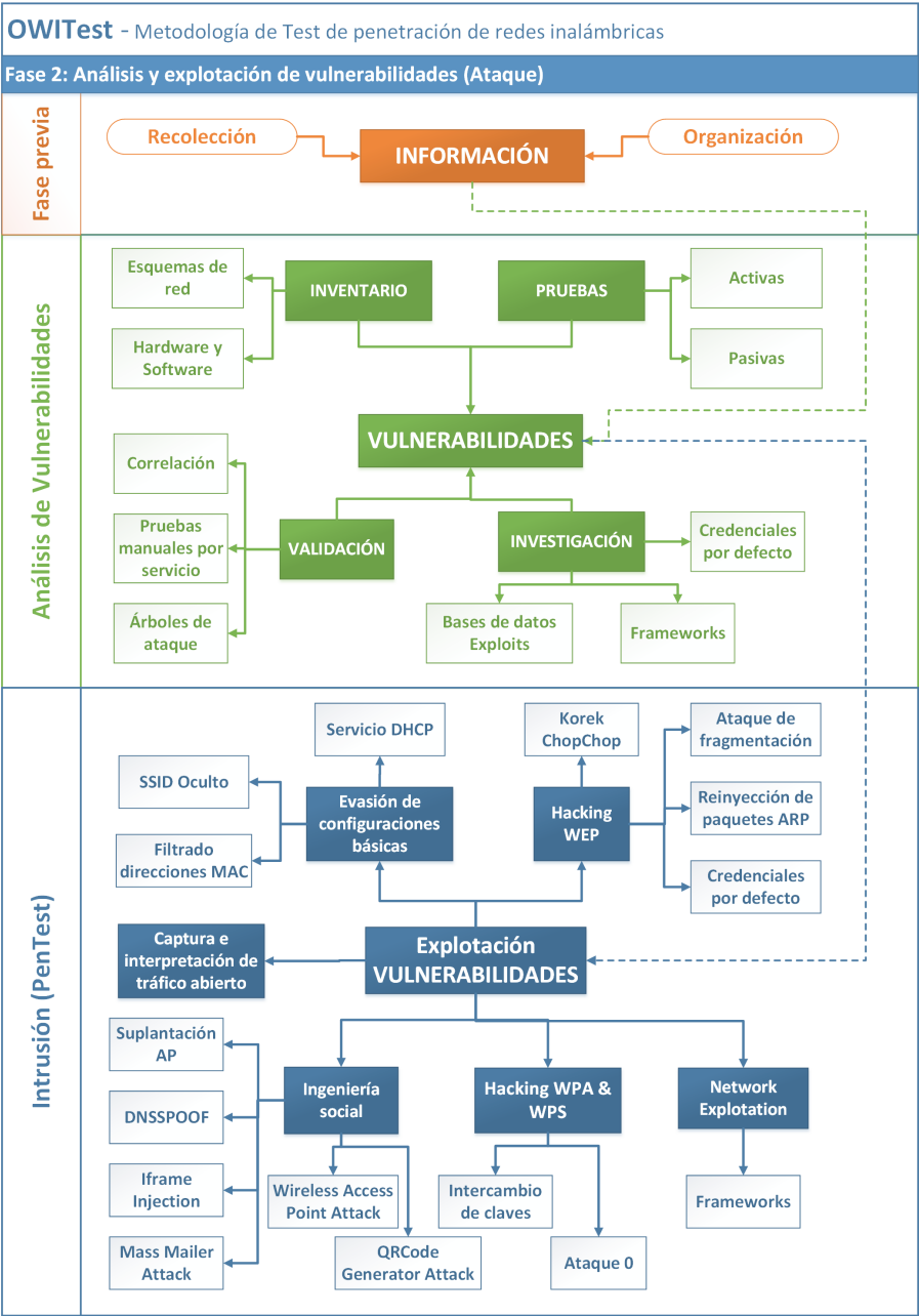
Figura 5 – Fase 2. Ataque (Narváez D., 2017)
