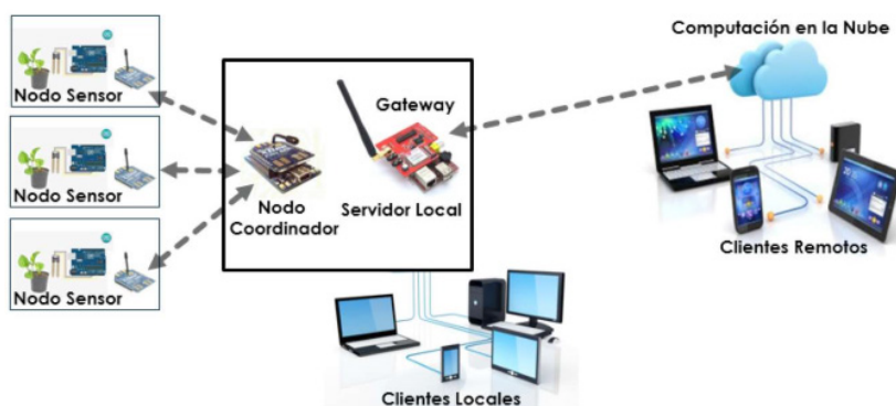
Figura 1 – Arquitectura del Sistema de Riego Autónomo basado en la Internet de las Cosas
