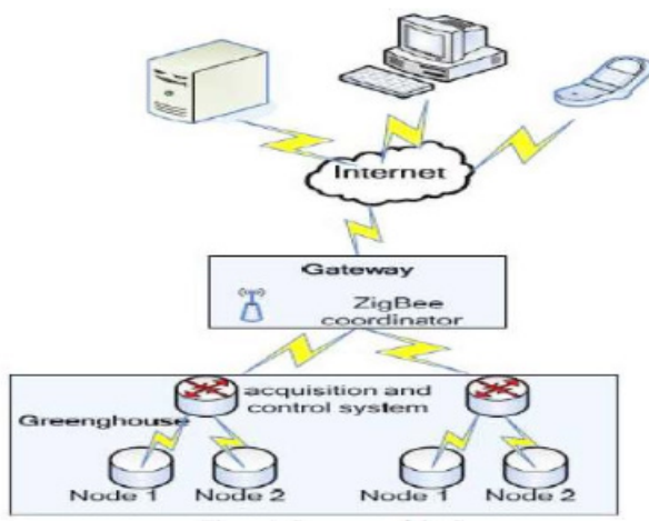
Figura 3 – Arquitectura del sistema inteligente de monitoreo de ambiente de invernaderos basado en el IoT.
