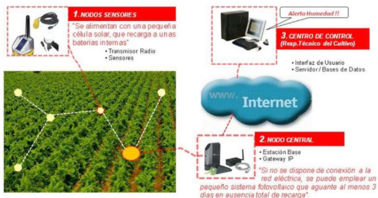
Figura 2 – Arquitectura Redes de Sensores sin Cables para Agricultura de Precisión en Regiones Minifundistas
