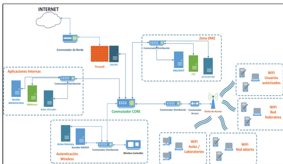
Figura 7 – Prototipo de validación (Narváez D., 2017)
