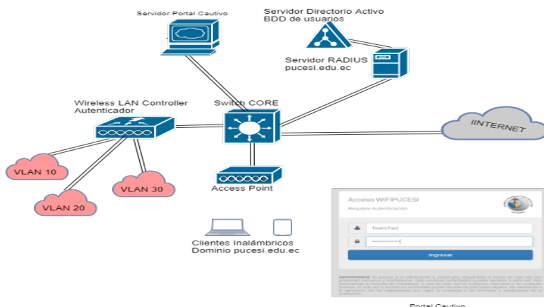
Figura 4 – Red Portal Cautivo (Sánchez E. Franklin, 2017)
