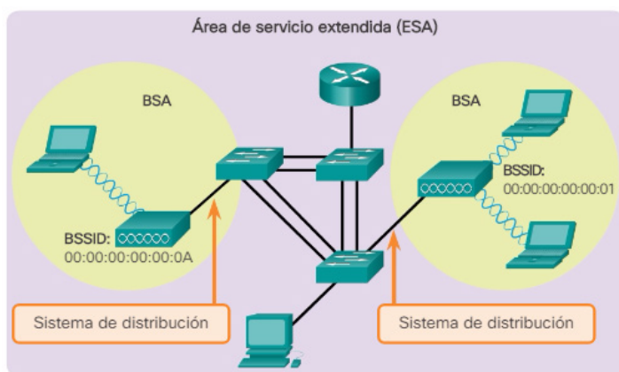
Figura 2 – Topología infraestructura (CISCO CCNA, 2016)
