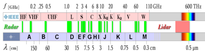
Figura 2 – Rangos de ondas y de frecuencias utilizadas por radares.
